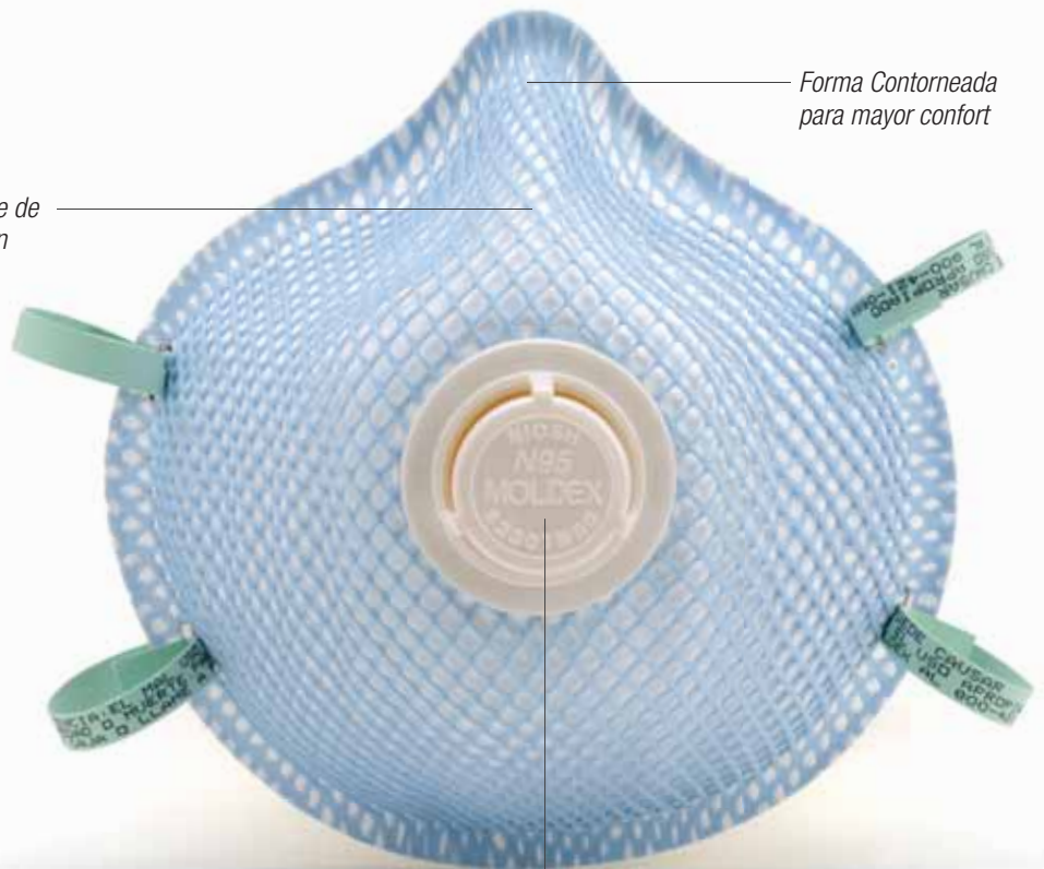
La malla Dura-Mesh interior previene el colapso por el calor y la humedad
